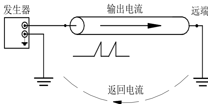
图 3 基本电路
